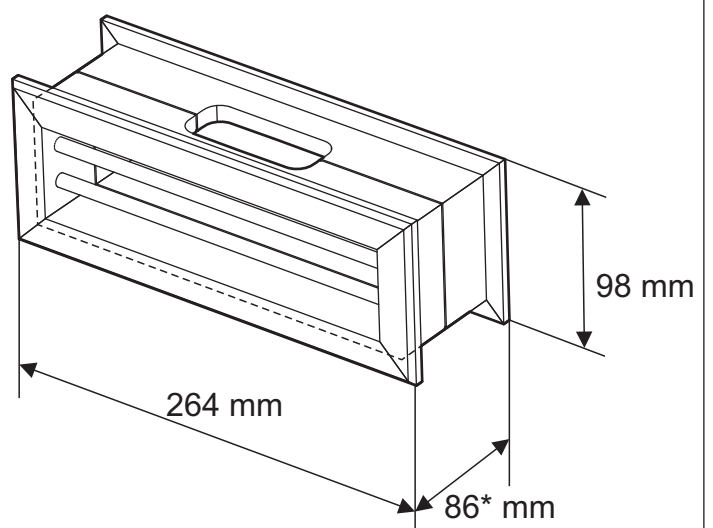
External dimensions Yttre mått
