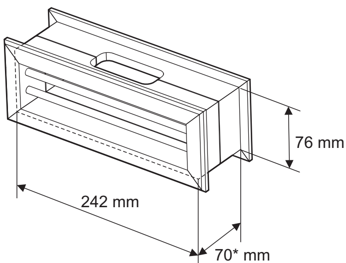
Dimensions for mounting Mått för montering
