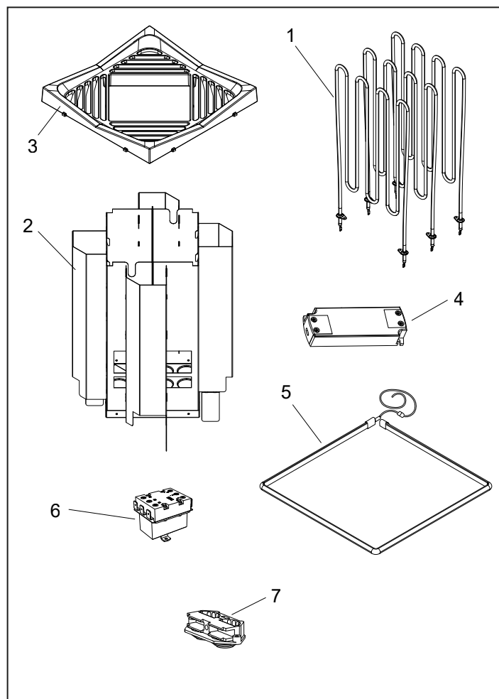
Rysunek 3. Części zamienne
