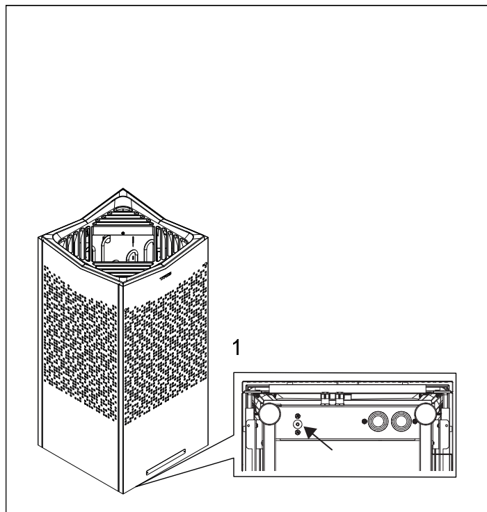
Illustration 2 : Réinitialisation de la protection thermique
