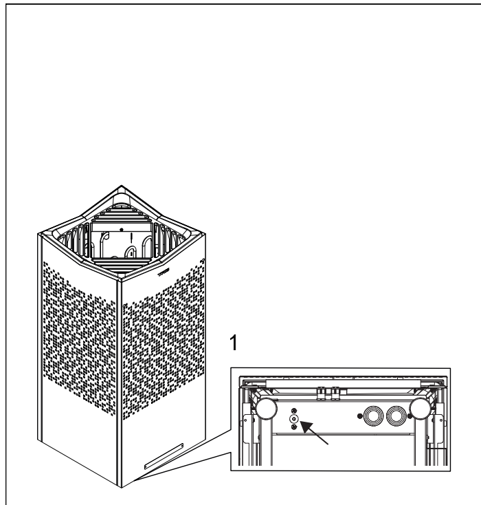
Afbeelding 2: De temperatuuruitschakeling resetten
