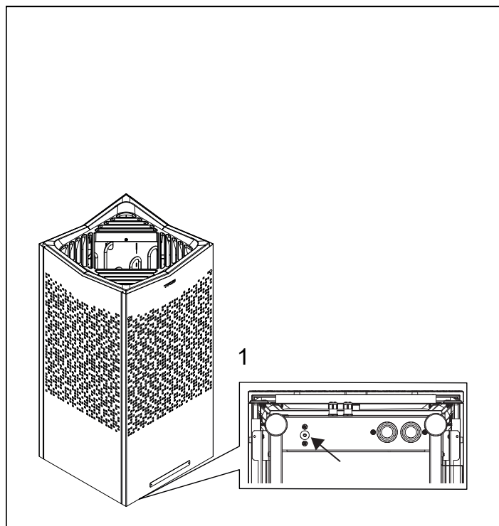
Fig 2: Återställning av temperaturskyddet.
