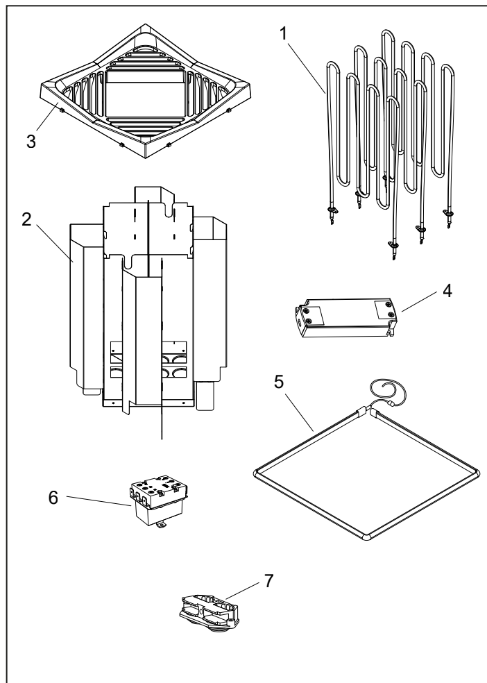
Abbildung 3: Ersatzteile
