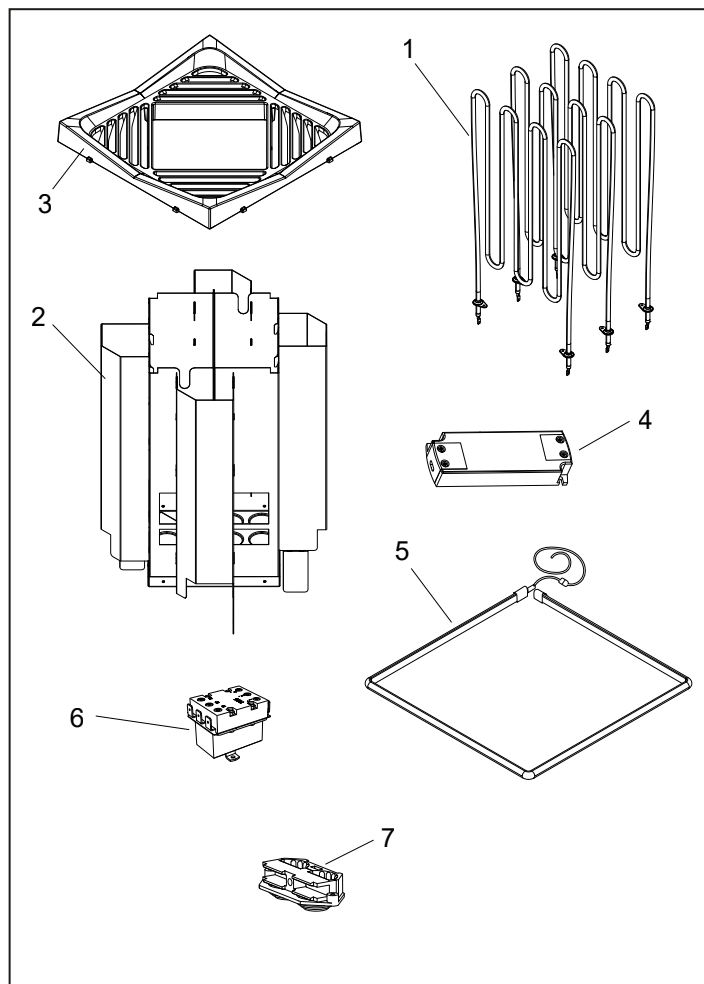
Illustration 3 : Pièces de rechange
