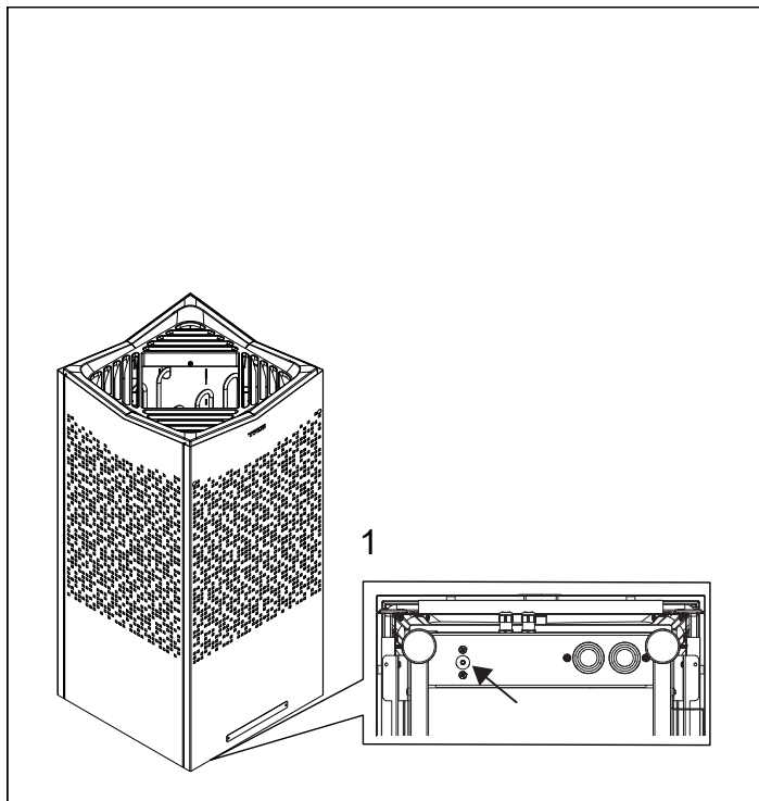
Rysunek 2. Resetowanie wyłącznika termicznego
