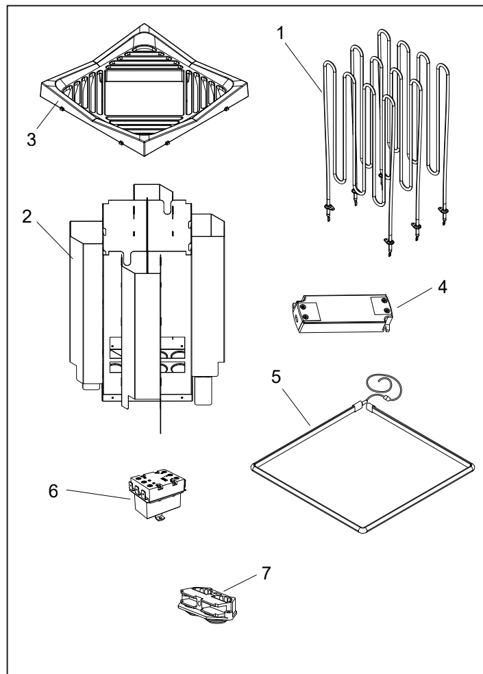
Fig 3: Reservdelar
