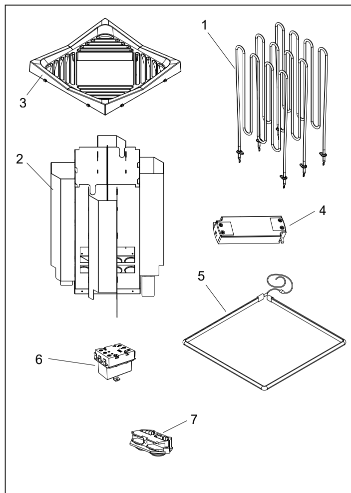
Afbeelding 3: Reserveonderdelen
