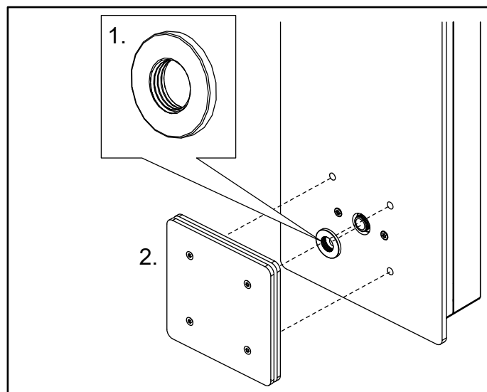
Afb. 17 1. Schroef de afdekring met de hand op zijn plaats zodat deze vlak tegen het glas aanligt. 2. Monteer het stoompijpje
