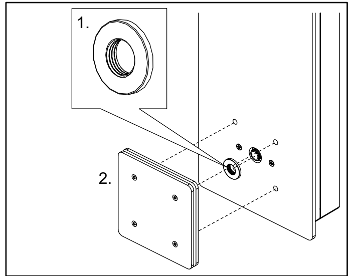
Kuva 17 1. Kierrä kannen aluslevy paikalleen käsin niin, että se on tasaisesti lasia vasten. 2. Asenna höyrystin
