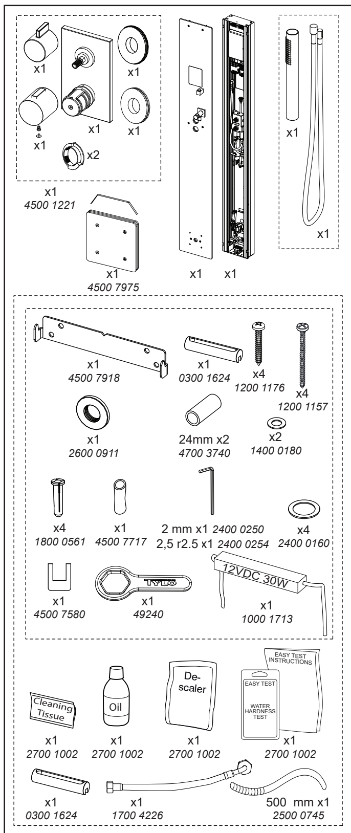
Kuva 1 Höyrypylvään osat
