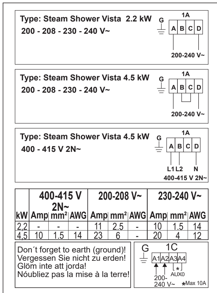
Abb 7. Anschlussplan
