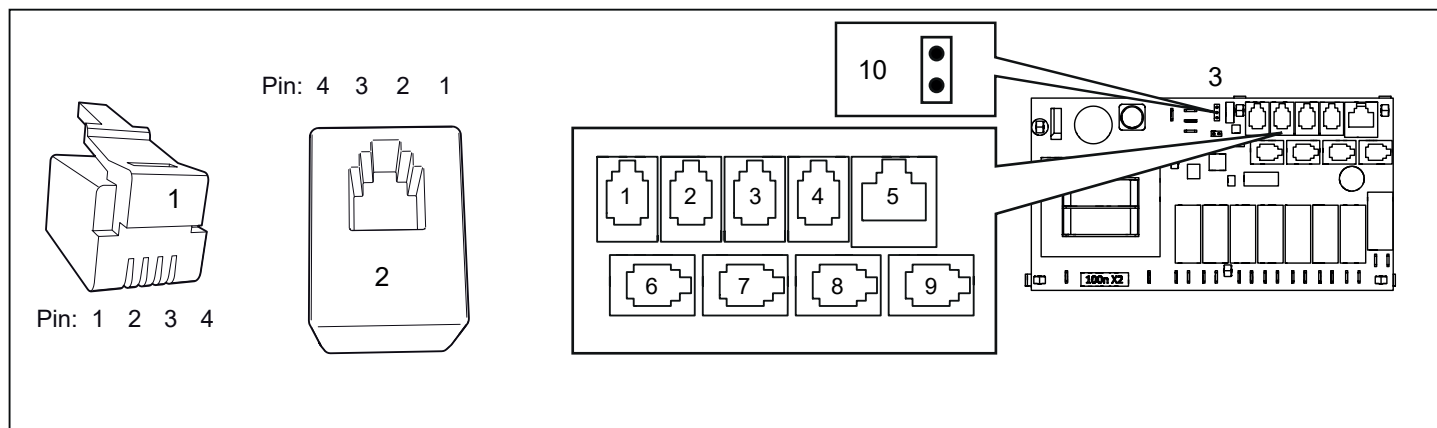
Abb. 10 Modularer Stecker/Schütz und Relaisplatine High
