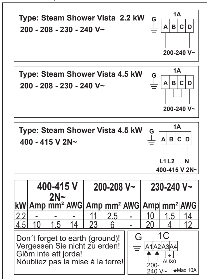
Рис. 7 Схема соединений
