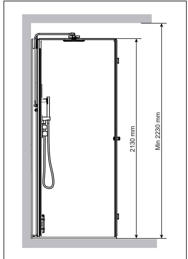
Fig. 2 Höjdmått Vista
