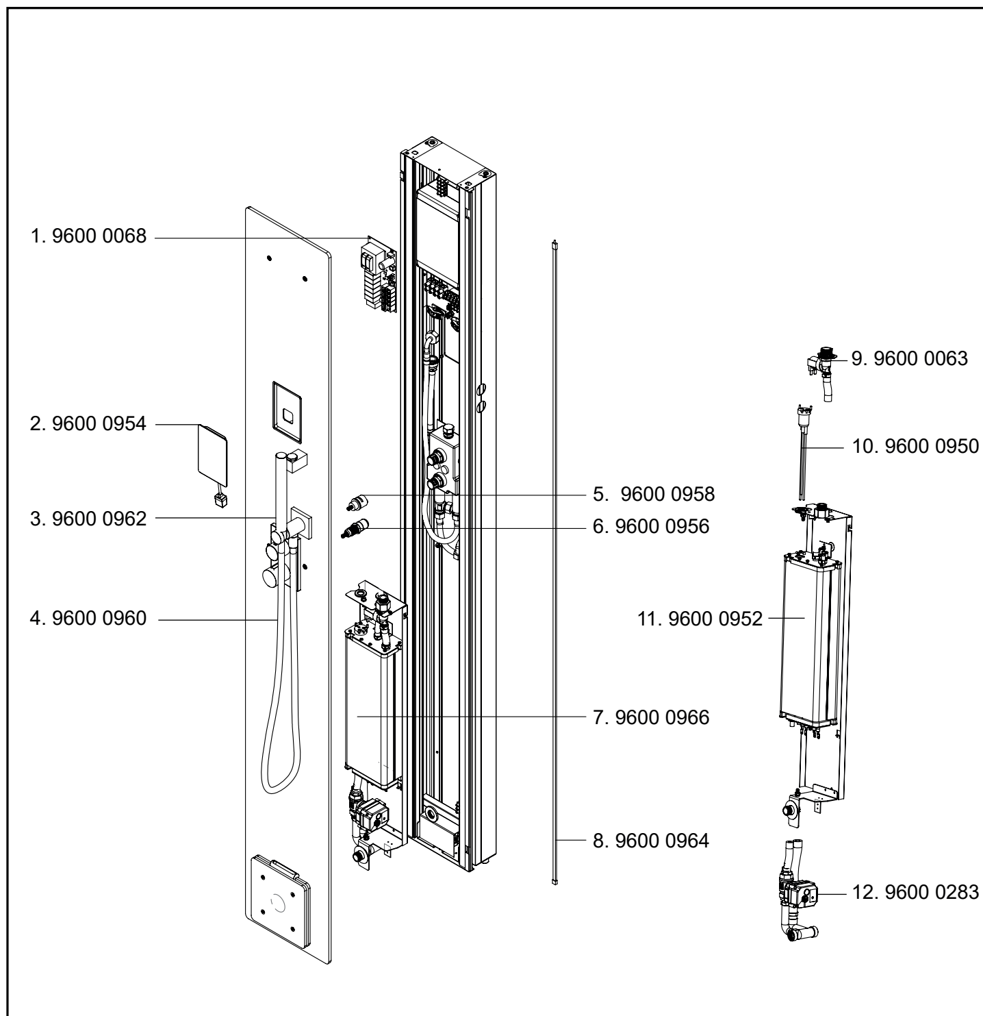
Afb. 11 Reserveonderdelen
