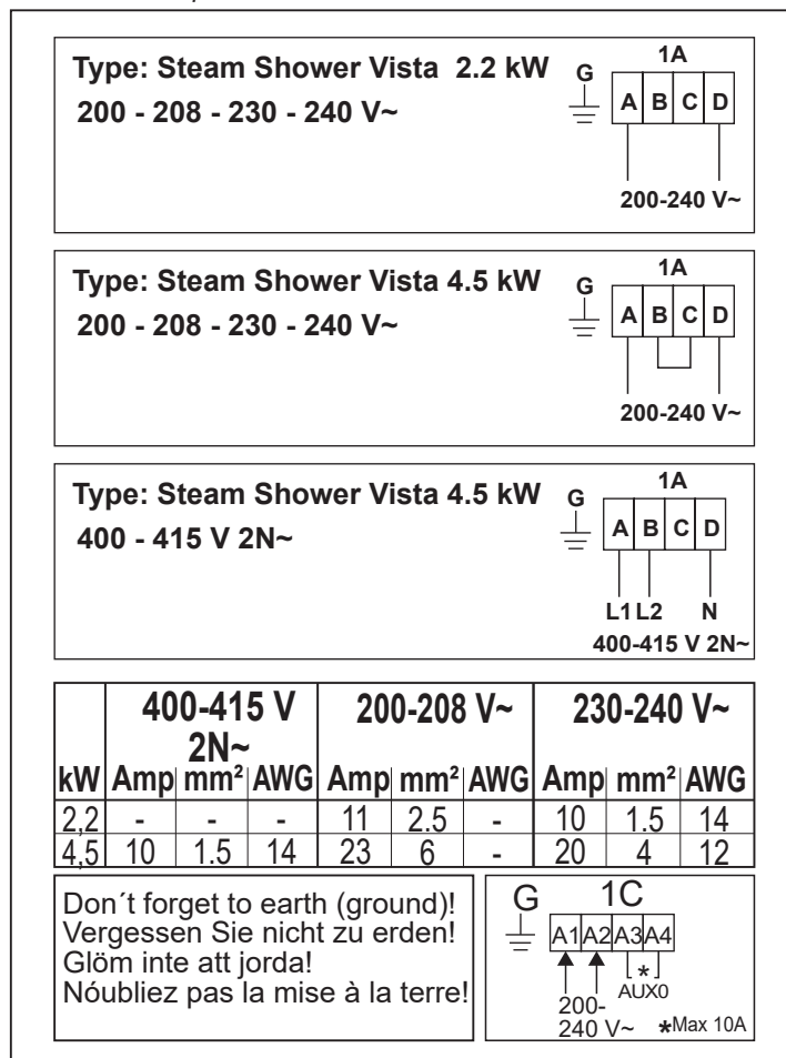
Figure 7 : Schéma de raccordement
