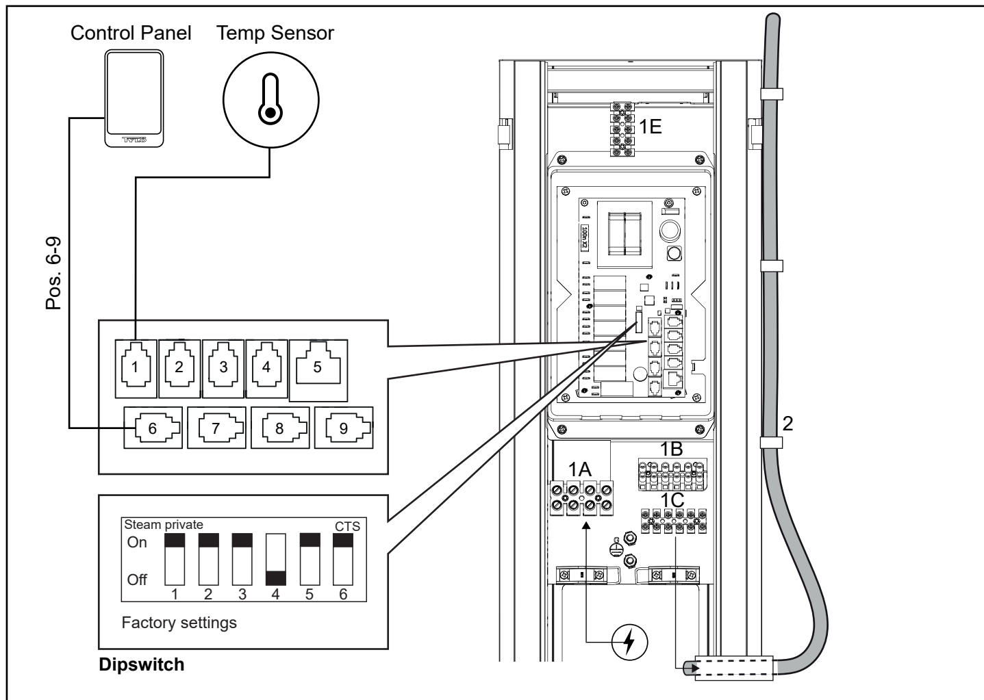
Kuva 5 Asennuksen kytkentäkaavio, Stella-höyrygeneraattori
