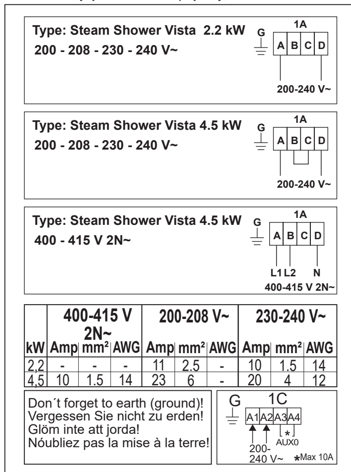
Rys. 7. Schemat połączeń.
