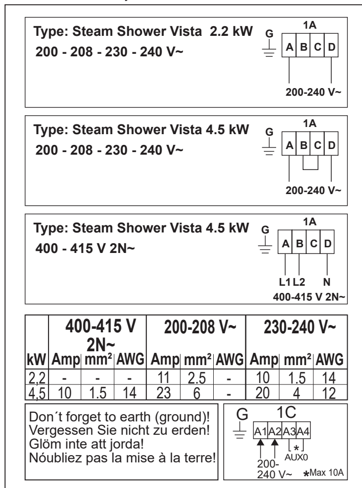
Fig. 7 Inkopplingsschema
