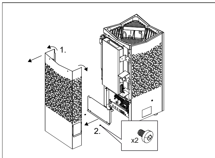
Illustration 10 : Retirez le capot arrière et la trappe inférieure.
